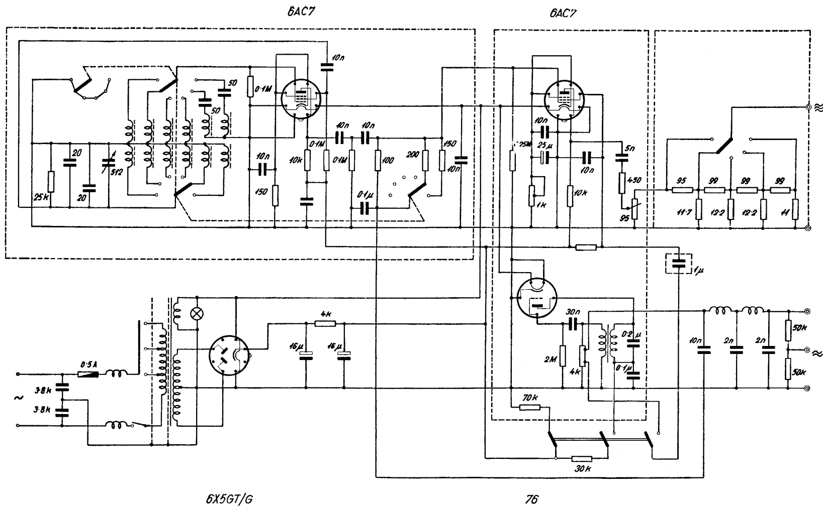
543. 67. ábra. Az EMG 1162 típusú üzemi rádiófrekvenciás áramforrás kapcsolási rajza
